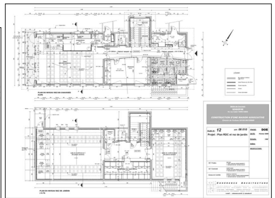
Plans d'origines qui ont été revus et corrigés, entre autres pour l'installation des placards
